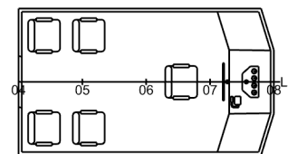
VISTA SUPERIOR (CABINA)
